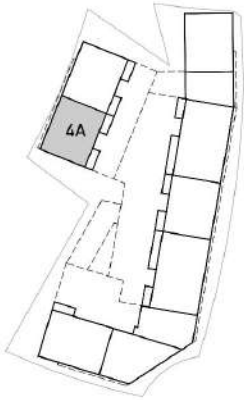
РАЗПРЕДЕЛЕНИЕ НИВО 2 НА КОТА +3.55, М1:100 | СГРАДА 4А
