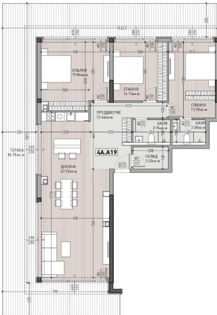
АПАРТАМЕНТ 19 НИВО 6 НА КОТА +15.71, М1:80 | СГРАДА 4А
