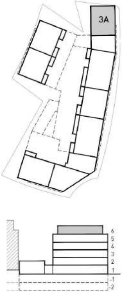
РАЗПРЕДЕЛЕНИЕ НИВО 6 НА КОТА +14.11, М1:100 | СГРАДА 3А
