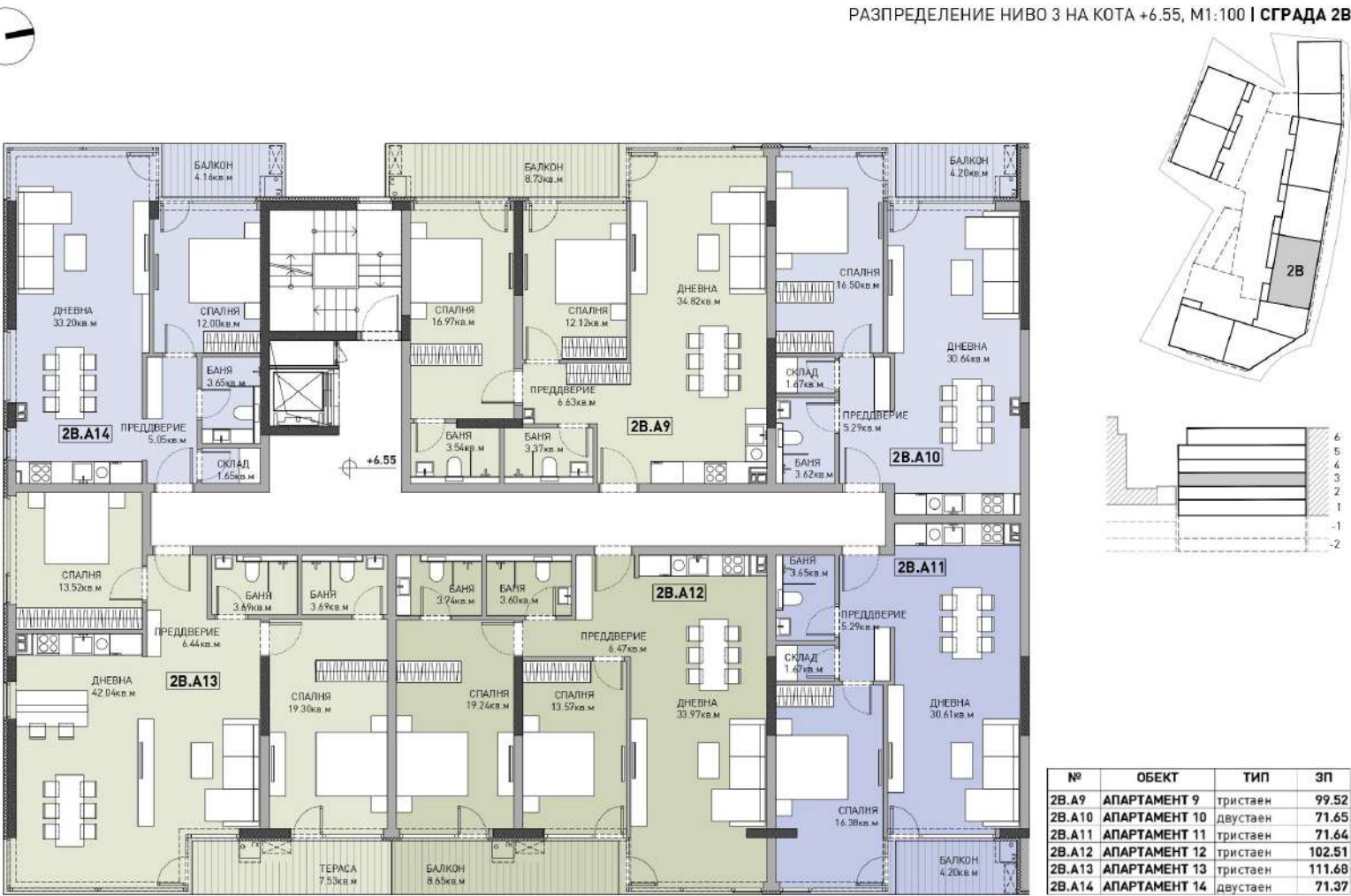
РАЗПРЕДЕЛЕНИЕ НИВО 3 НА КОТА +6.55, М1:100 | СГРАДА 2В
