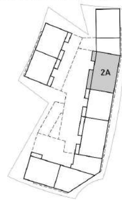
РАЗПРЕДЕЛЕНИЕ НИВО 1 НА КОТА ±0.00, М1:100 | СГРАДА 2А
