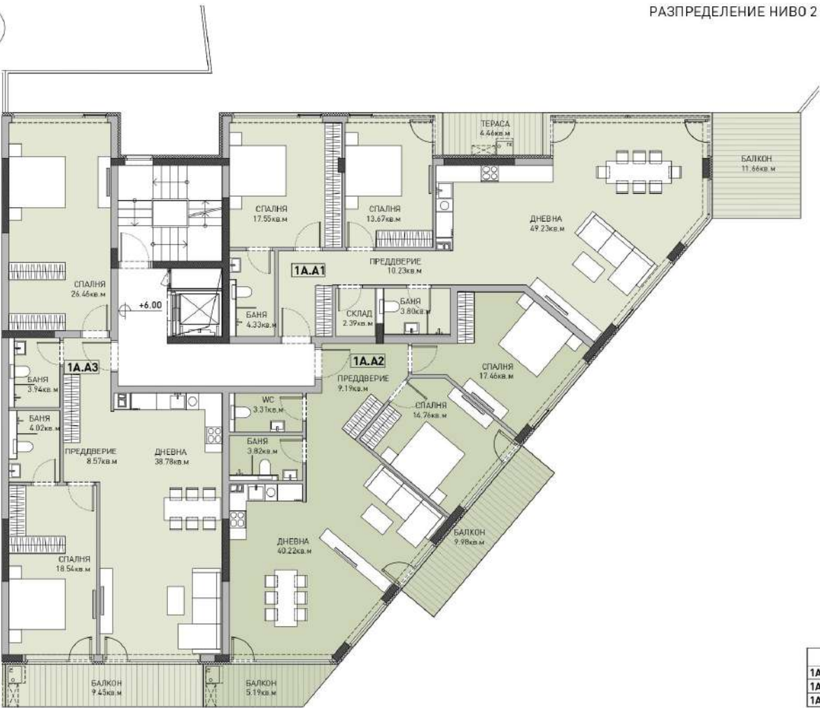
РАЗПРЕДЕЛЕНИЕ НИВО 2 НА КОТА +6.00, М1:100 | СГРАДА 1А
