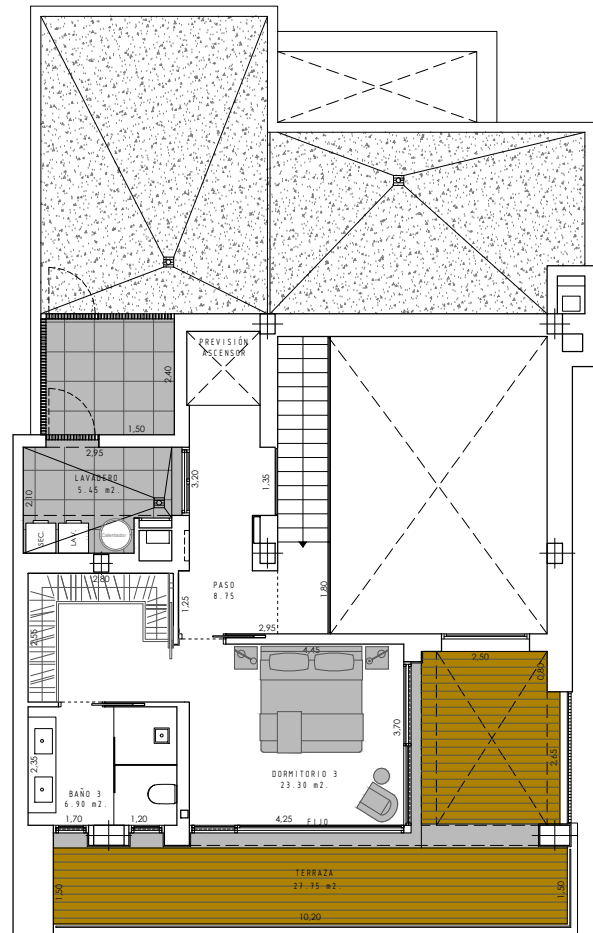
PLANTA ALTA
