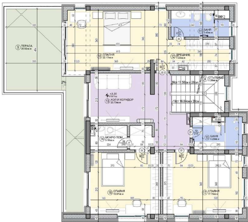
ЕДНОФАМИЛНА ЖИЛ. СГРАДА ТИП АЗ, РАЗПРЕДЕЛЕНИЕ КОТА +3.00
