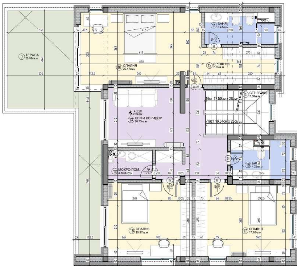
ЕДНОФАМИЛНА ЖИЛ. СГРАДА ТИП А2, РАЗПРЕДЕЛЕНИЕ КОТА +3.00
