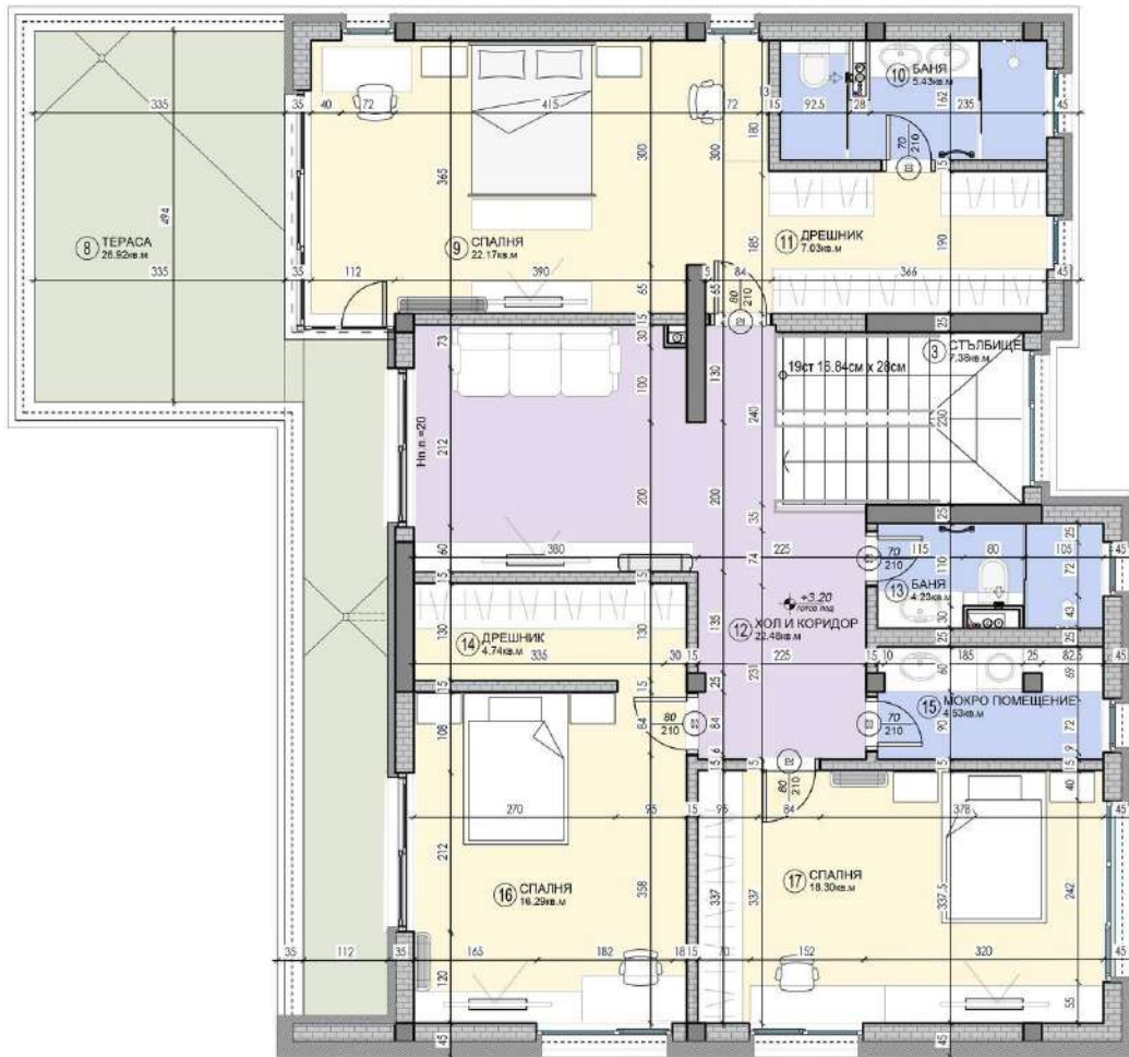
ЕДНОФАМИЛНА ЖИЛ. СГРАДА ТИП А1, РАЗПРЕДЕЛЕНИЕ КОТА +3.00
