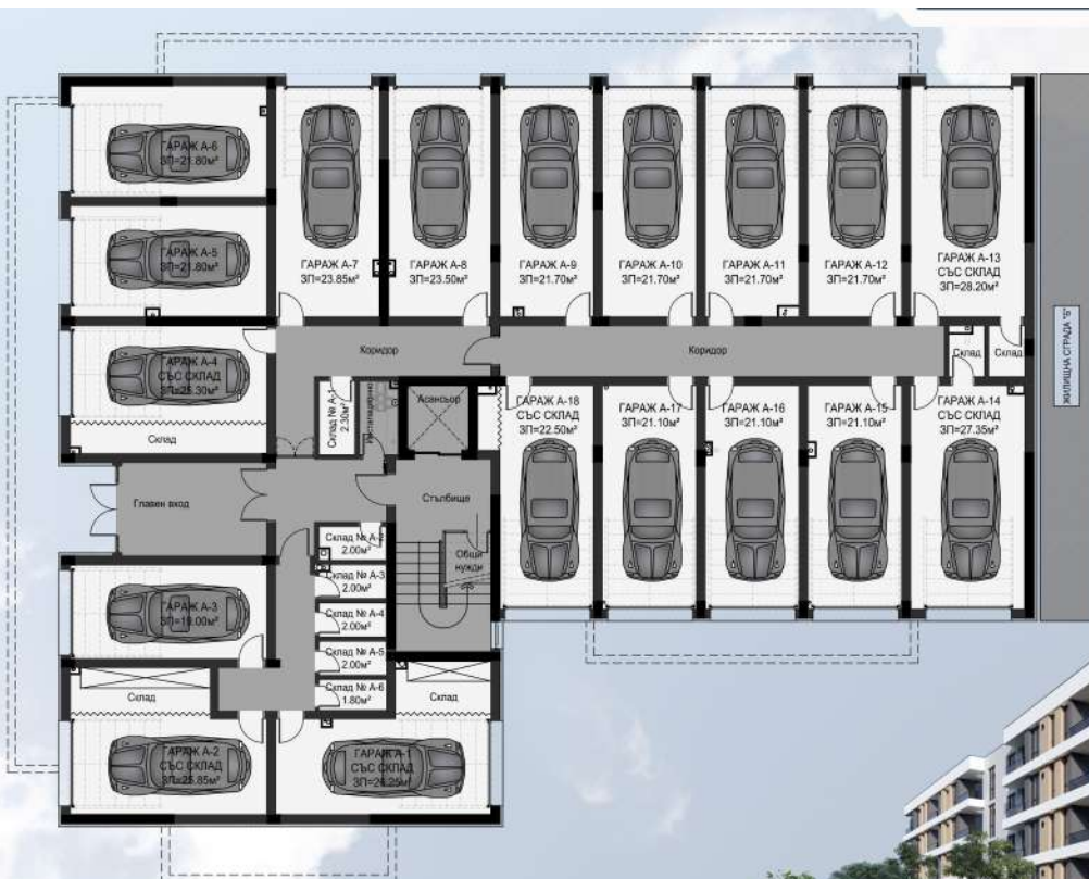
РАЗПРЕДЕЛЕНИЕ ПАРТЕРЕН ЕТАЖ МНОГОФАМИЛНА ЖИЛИЩНА СГРАДА "А"
