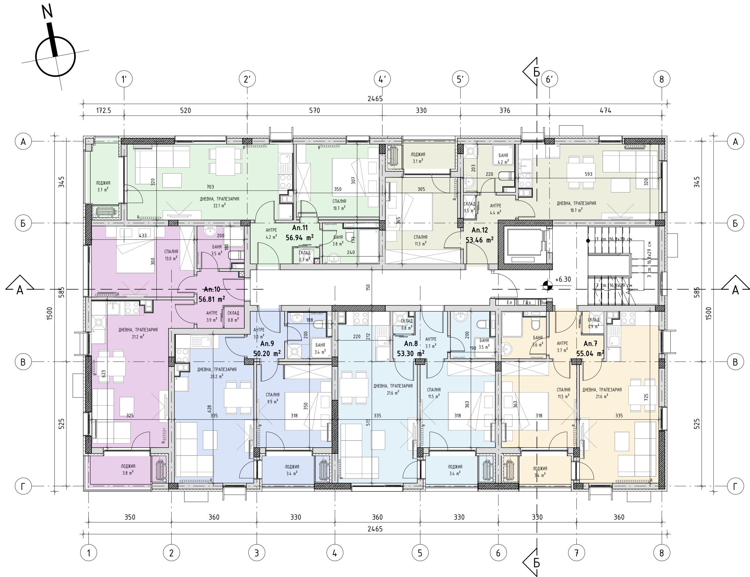
РАЗПРЕДЕЛЕНИЕ КОТА +6.30
