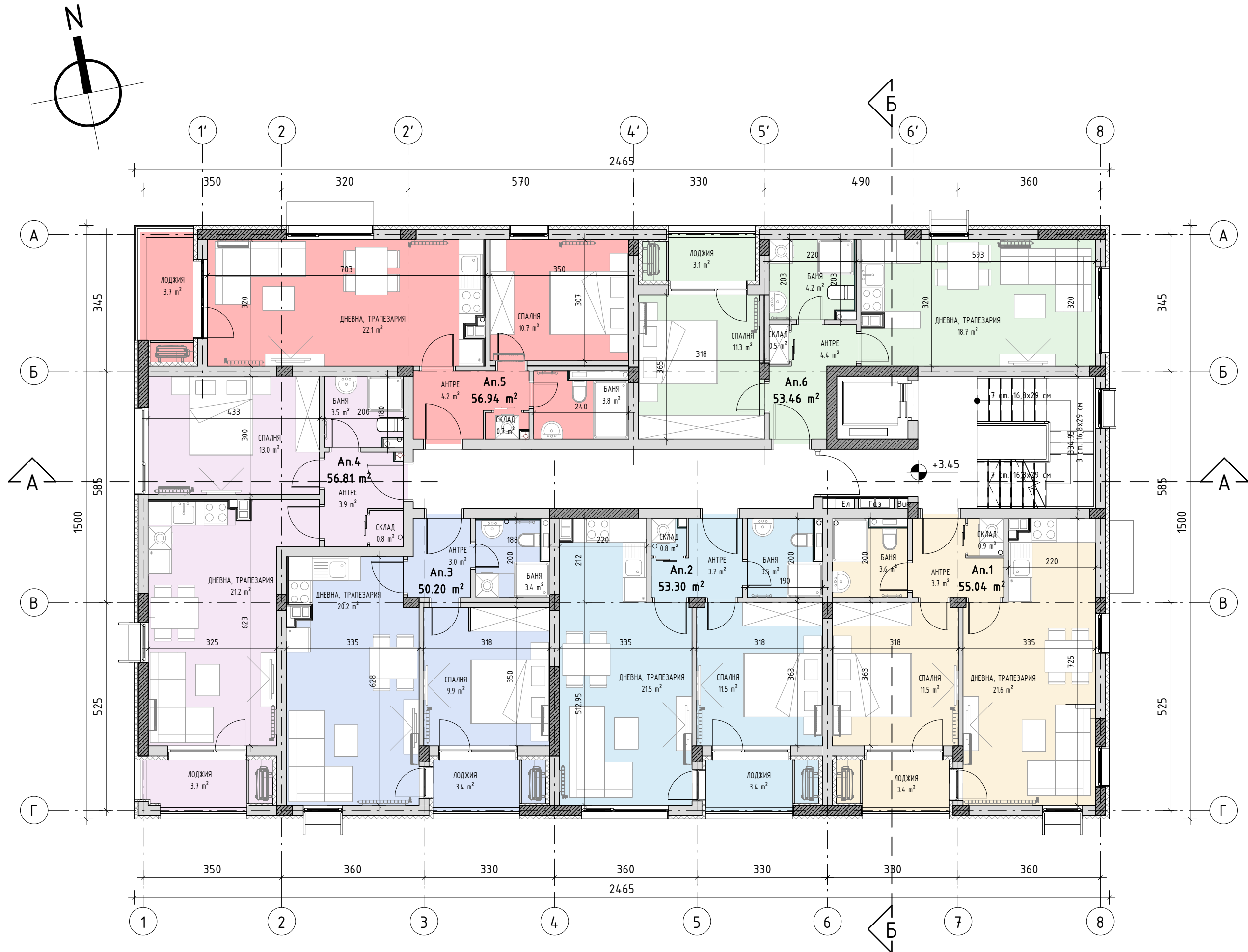
РАЗПРЕДЕЛЕНИЕ КОТА +3.45
