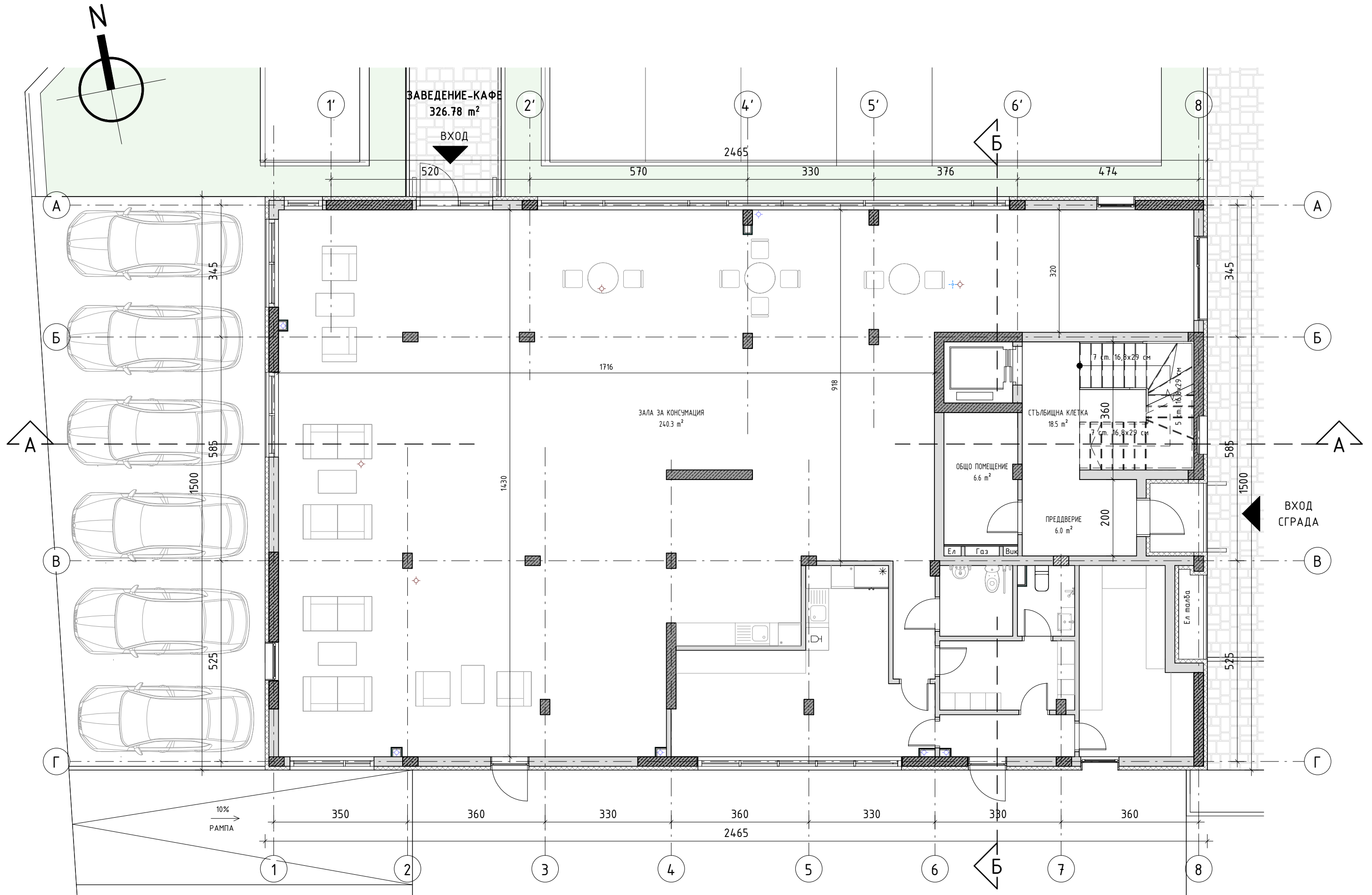
РАЗПРЕДЕЛЕНИЕ КОТА +0.00
