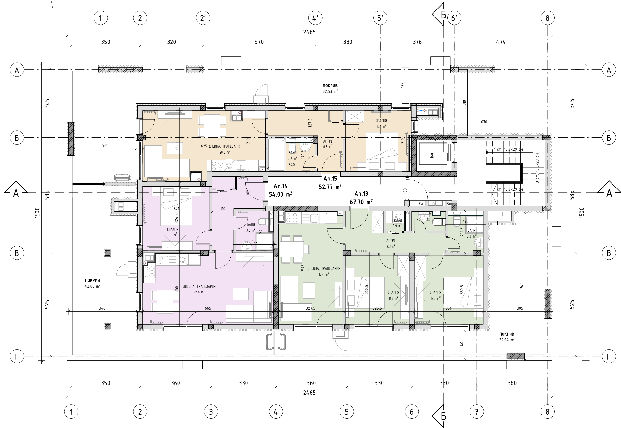
РАЗПРЕДЕЛЕНИЕ КОТА +9.15
