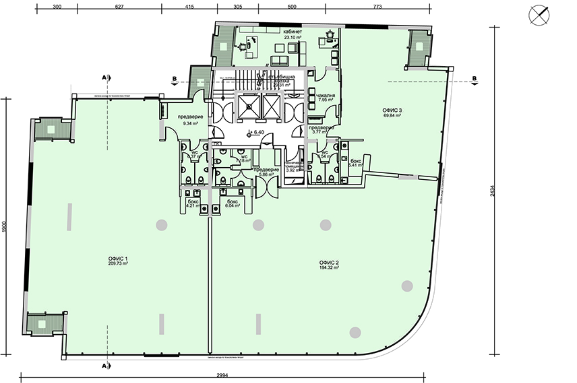
РАЗПРЕДЕЛЕНИЕ + 6.40; НИВО 3 ПЛОЩ НА ЕТАЖА - 666.67 m 2
