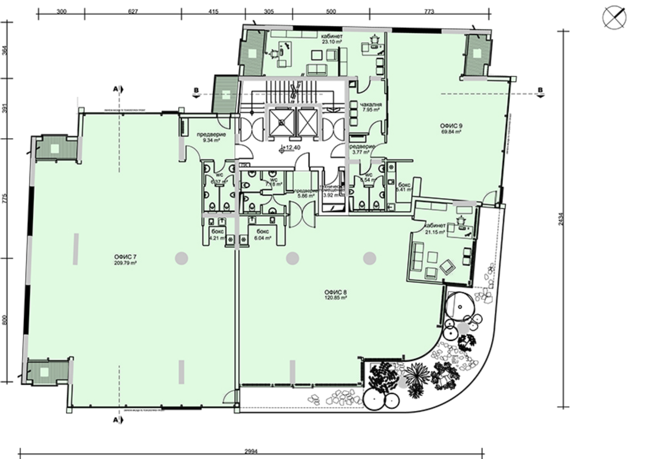
РАЗПРЕДЕЛЕНИЕ + 12.40; НИВО 5 ПЛОЩ НА ЕТАЖА - 674.97 m²
