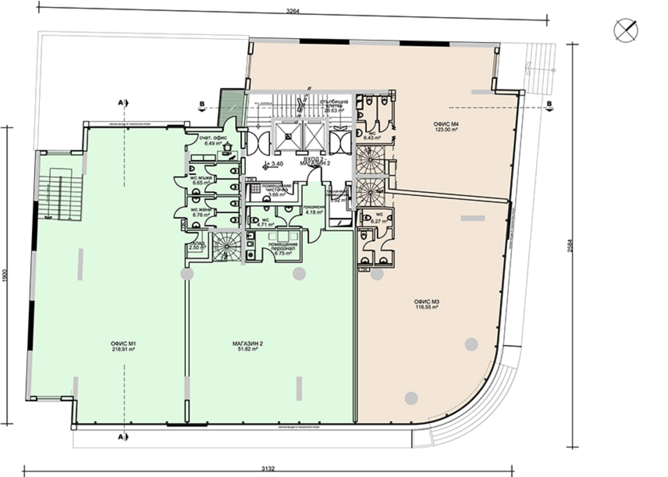
РАЗПРЕДЕЛЕНИЕ + 3.40; НИВО 2 ПЛОЩ НА ЕТАЖА - 682.36 m²
