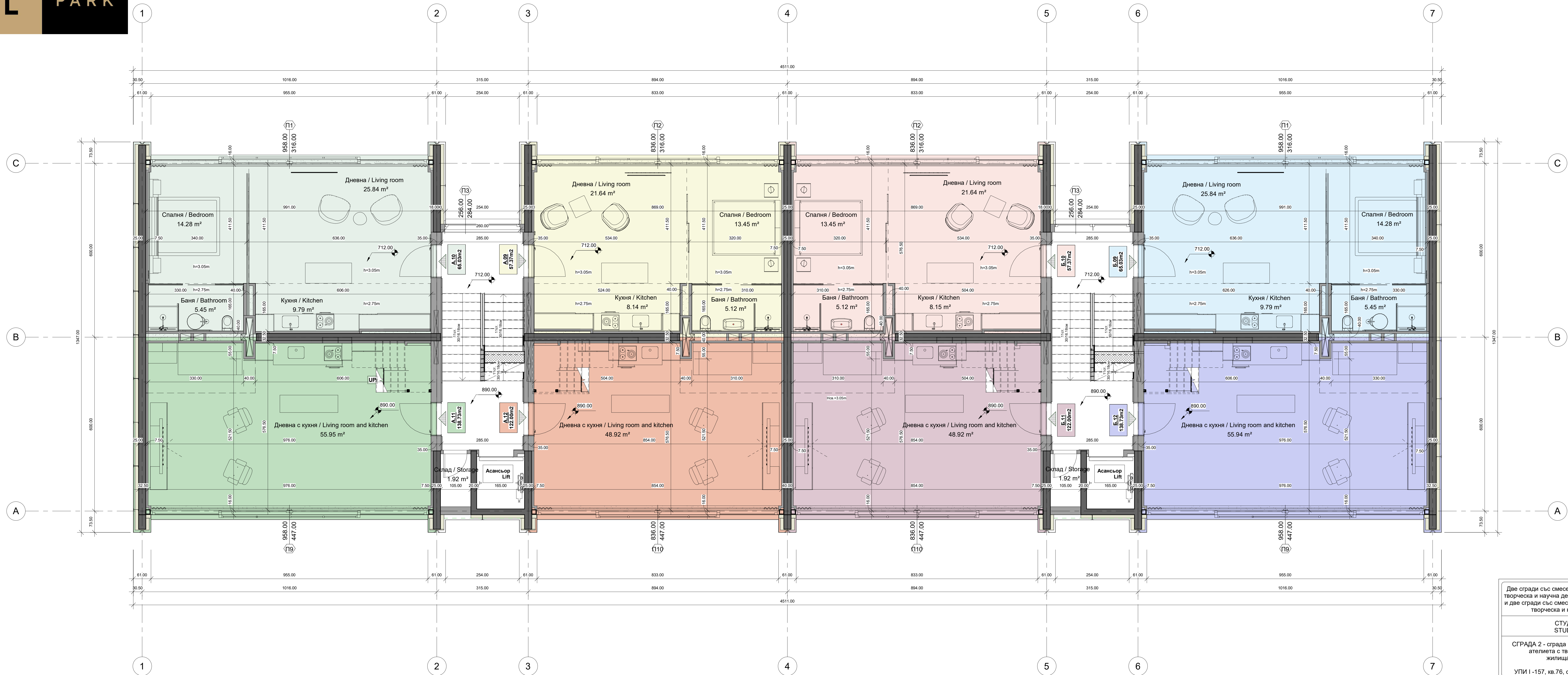
СГРАДА 2, ЕТАЖ 3 НИВО +7.12m / НИВО +8.90m BUILDING 2, FLOOR 3 LEVEL +7.12m / LEVEL +8.90m
