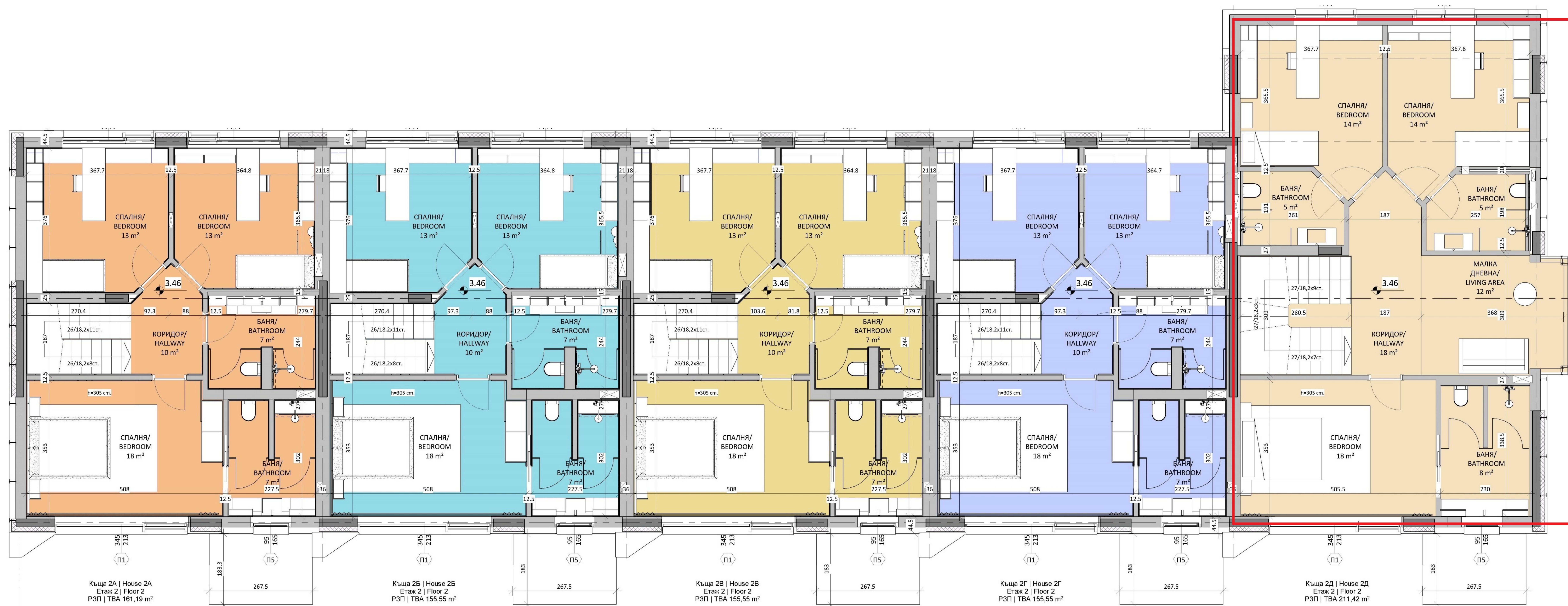
Къща 2А | House 2A РЗП | ТВА 161,19 m 2
