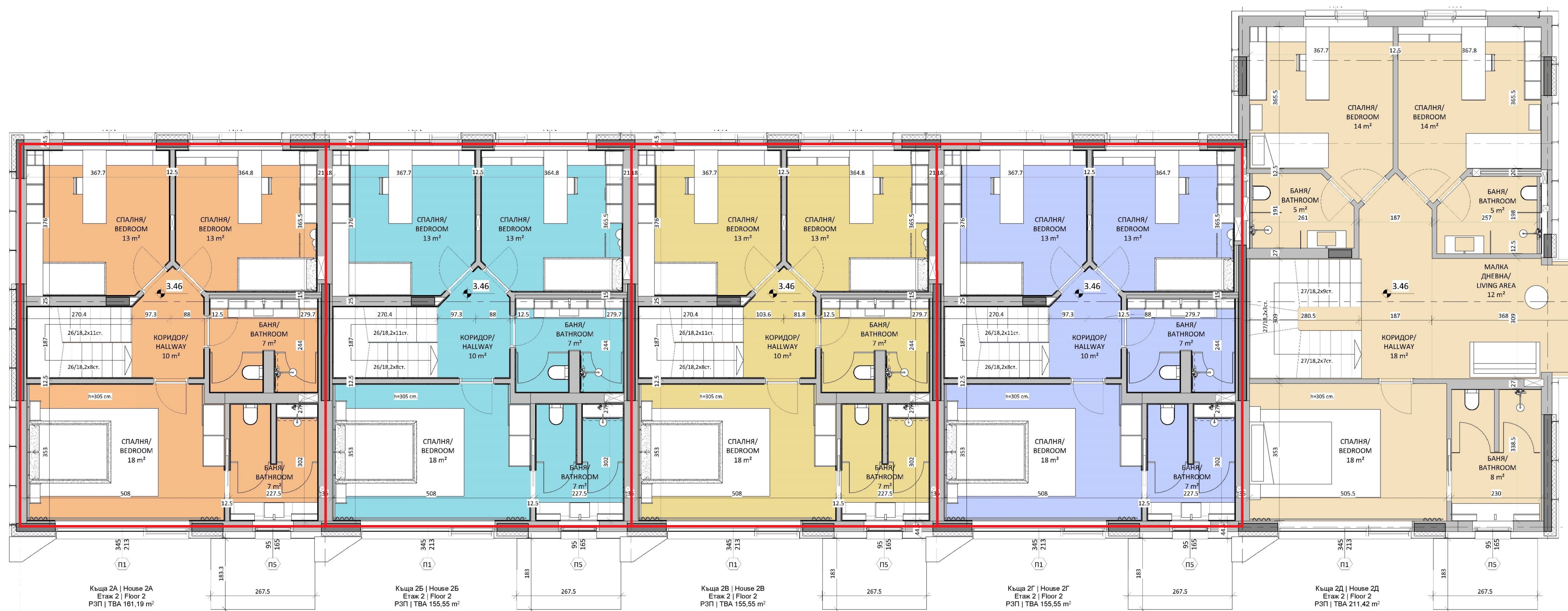
Къща 2А | House 2А РЗП | ТВА 161,19 m 2
