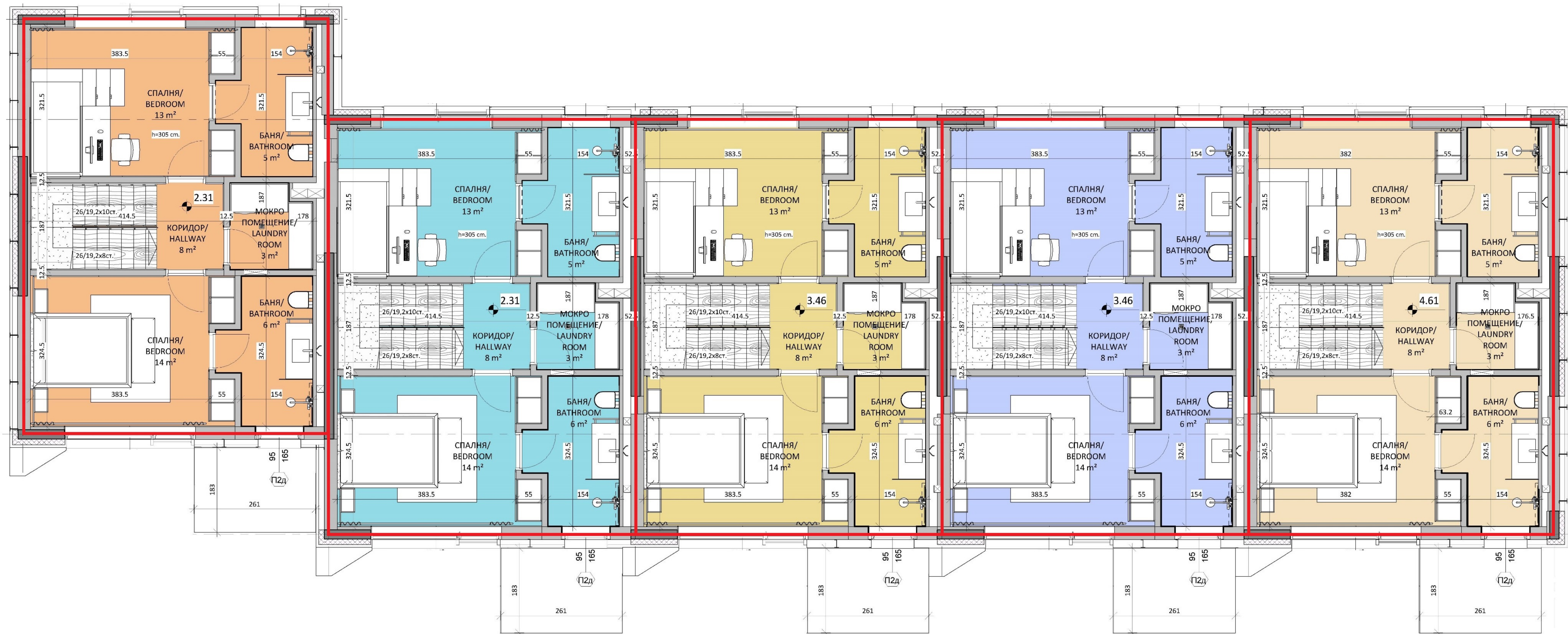
Къща 1А | House 1A РЗП | ТВА 128,97 m 2
