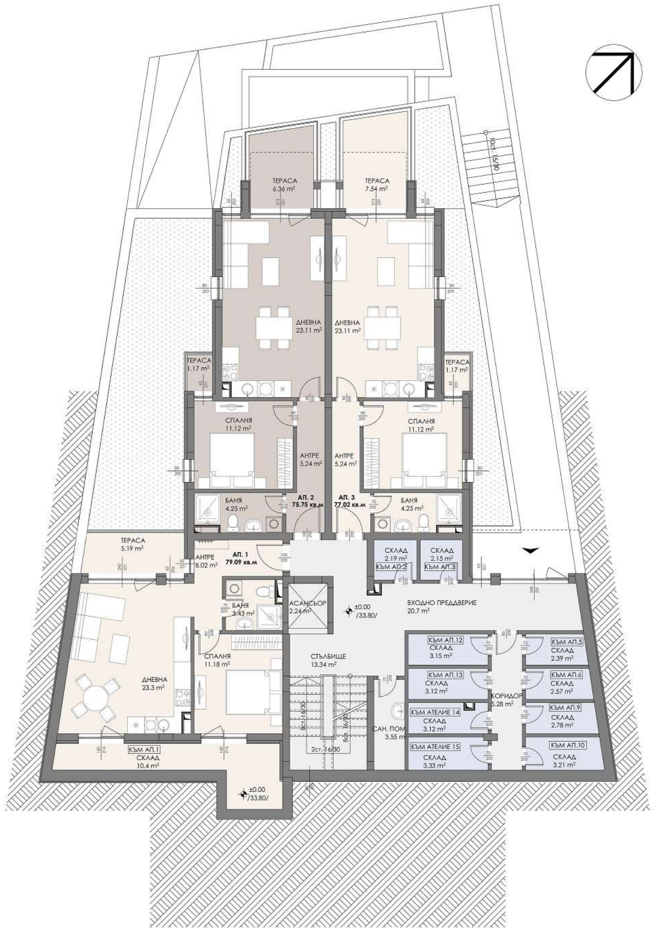
РАЗПРЕДЕЛЕНИЕ ±0,00 ПАРТЕР
