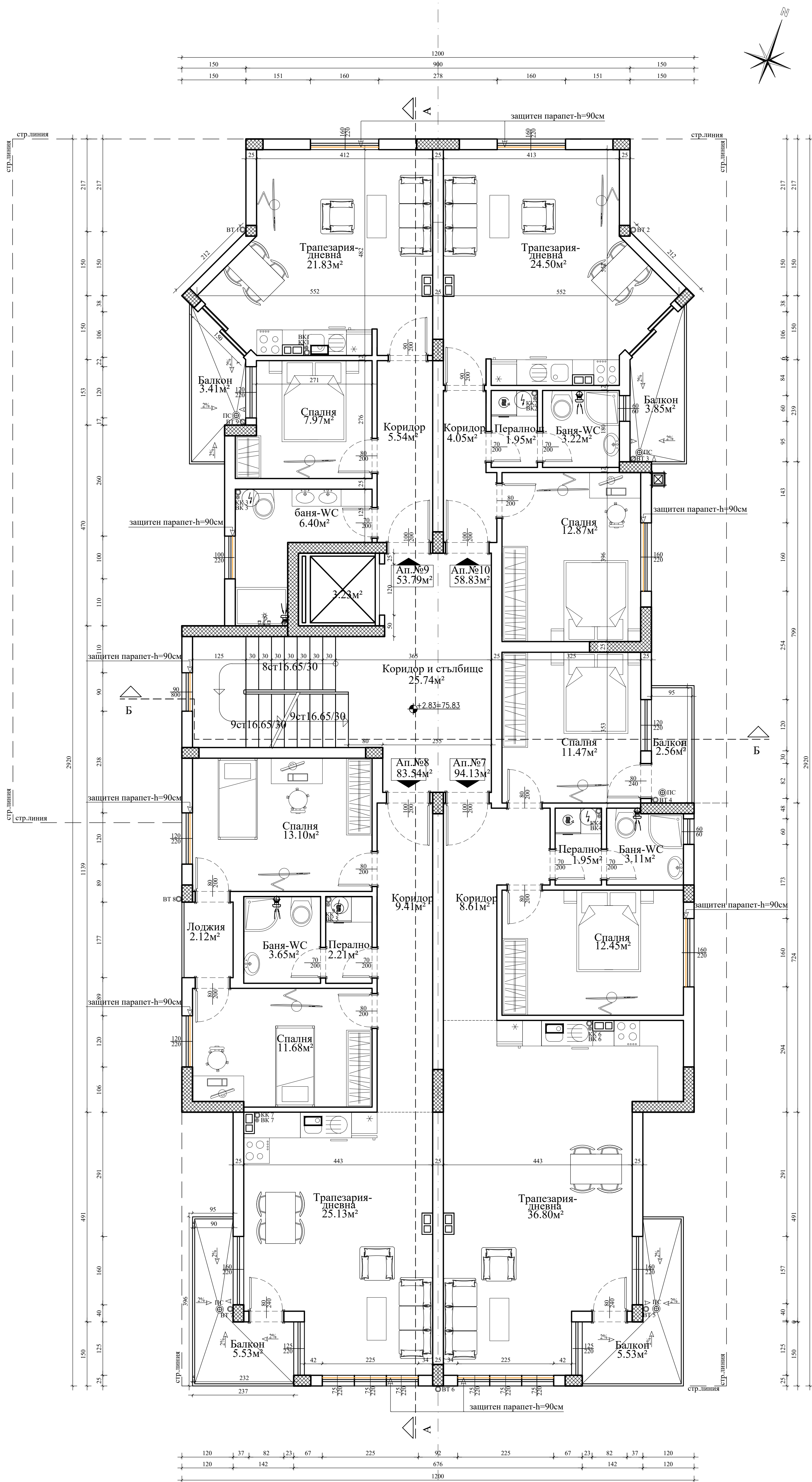
РАЗПРЕДЕЛЕНИЕ ВТОРИ ЕТАЖ КОТА +2.83
