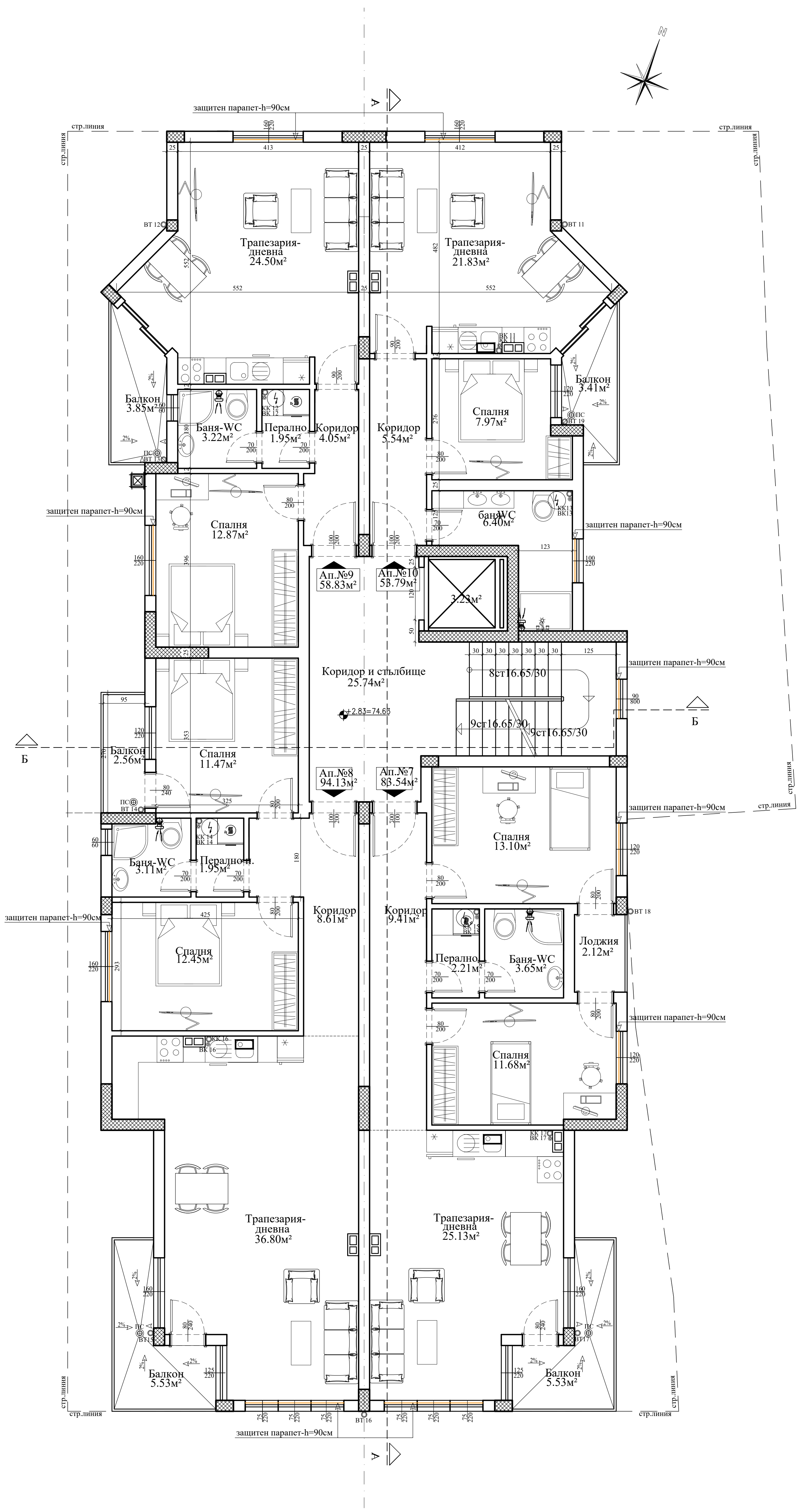
РАЗПРЕДЕЛЕНИЕ ВТОРИ ЕТАЖ КОТА +2.83
