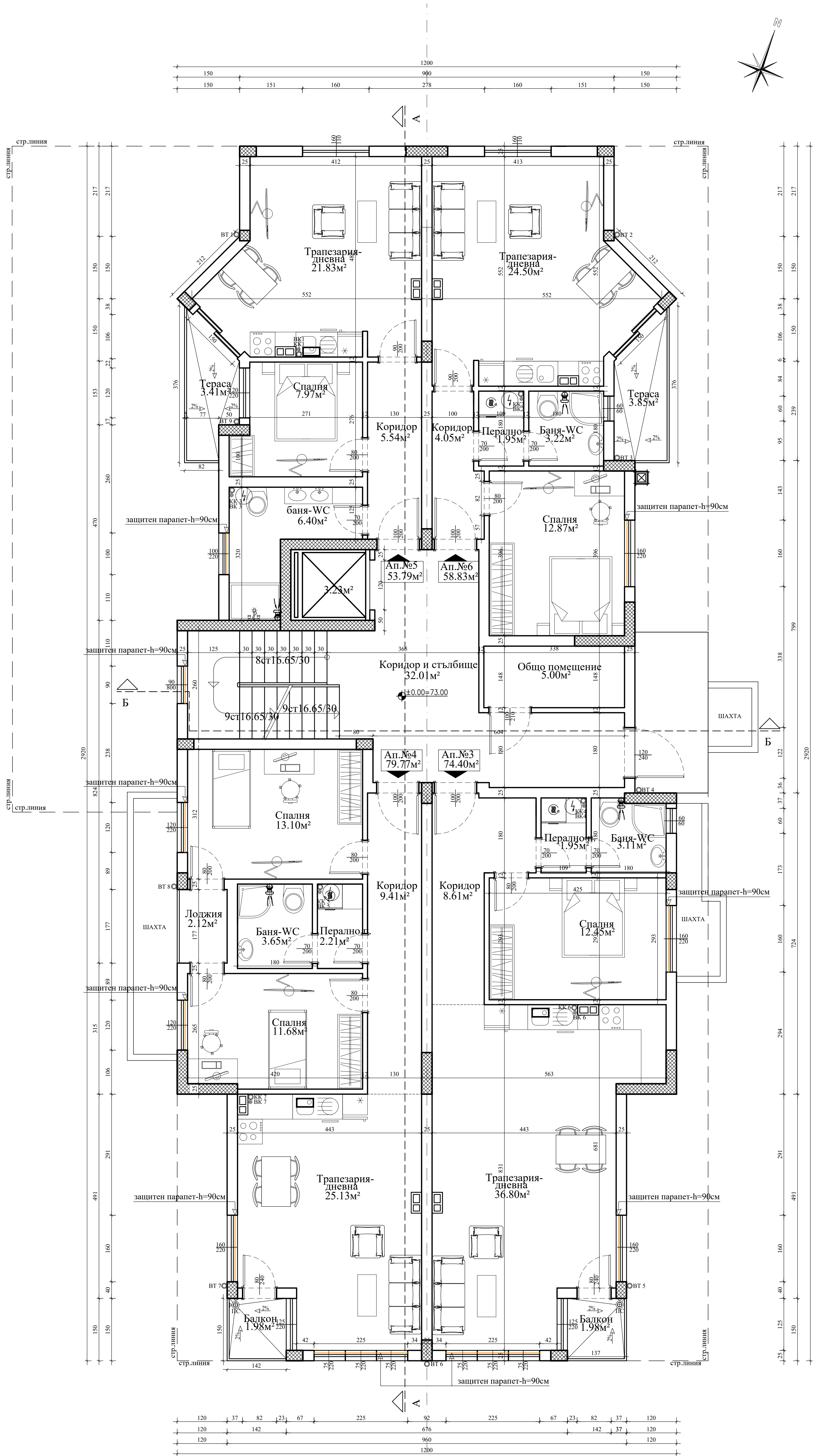
РАЗПРЕДЕЛЕНИЕ ПЪРВИ ЕТАЖ КОТА ±0.00
