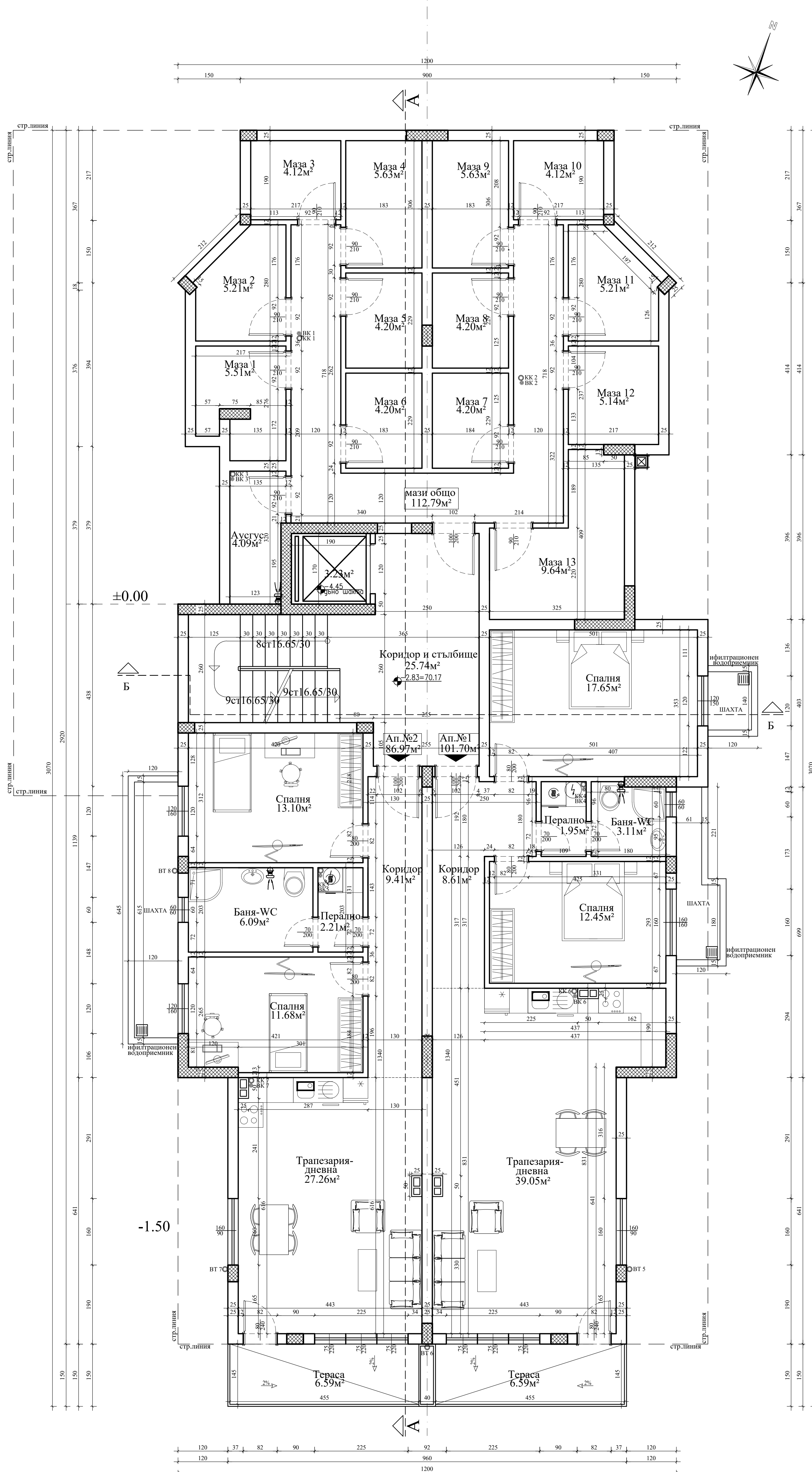
РАЗПРЕДЕЛЕНИЕ ПОЛУПОДЗЕМЕН ЕТАЖ- КОТА -2.83
