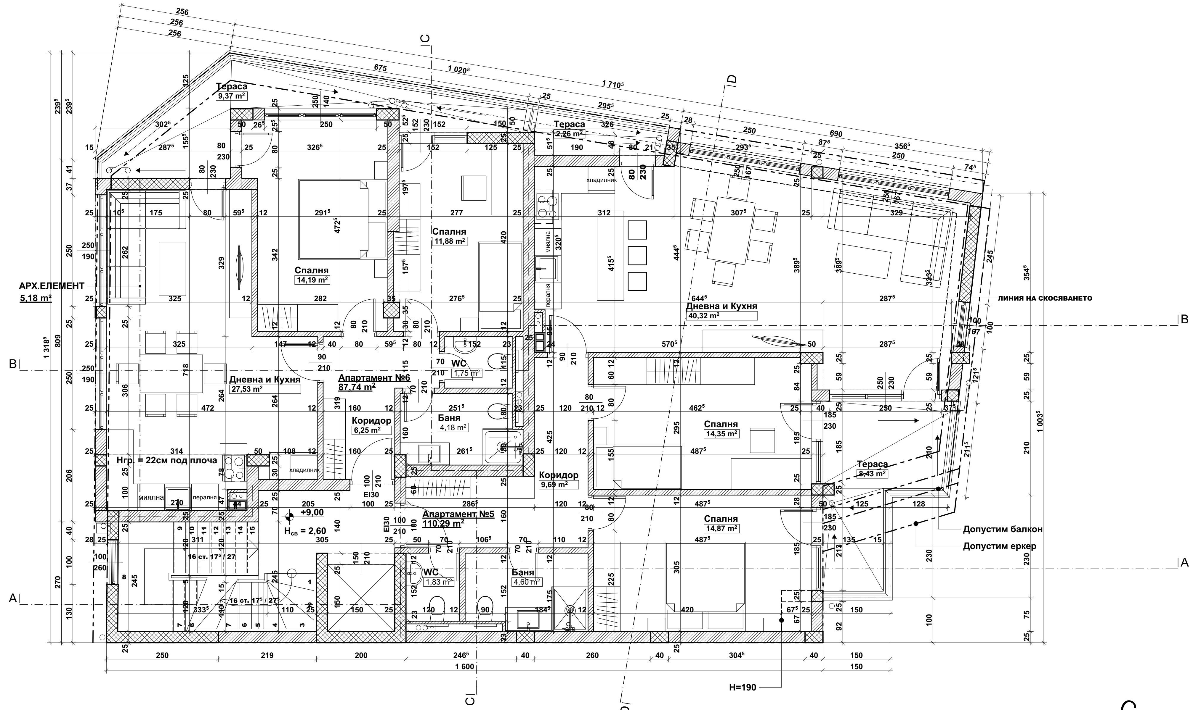
РАЗПРЕДЕЛЕНИЕ ТРЕТИ ЖИЛИЩЕН ЕТАЖ М 1:50 ЗП - 220,03 m 2
