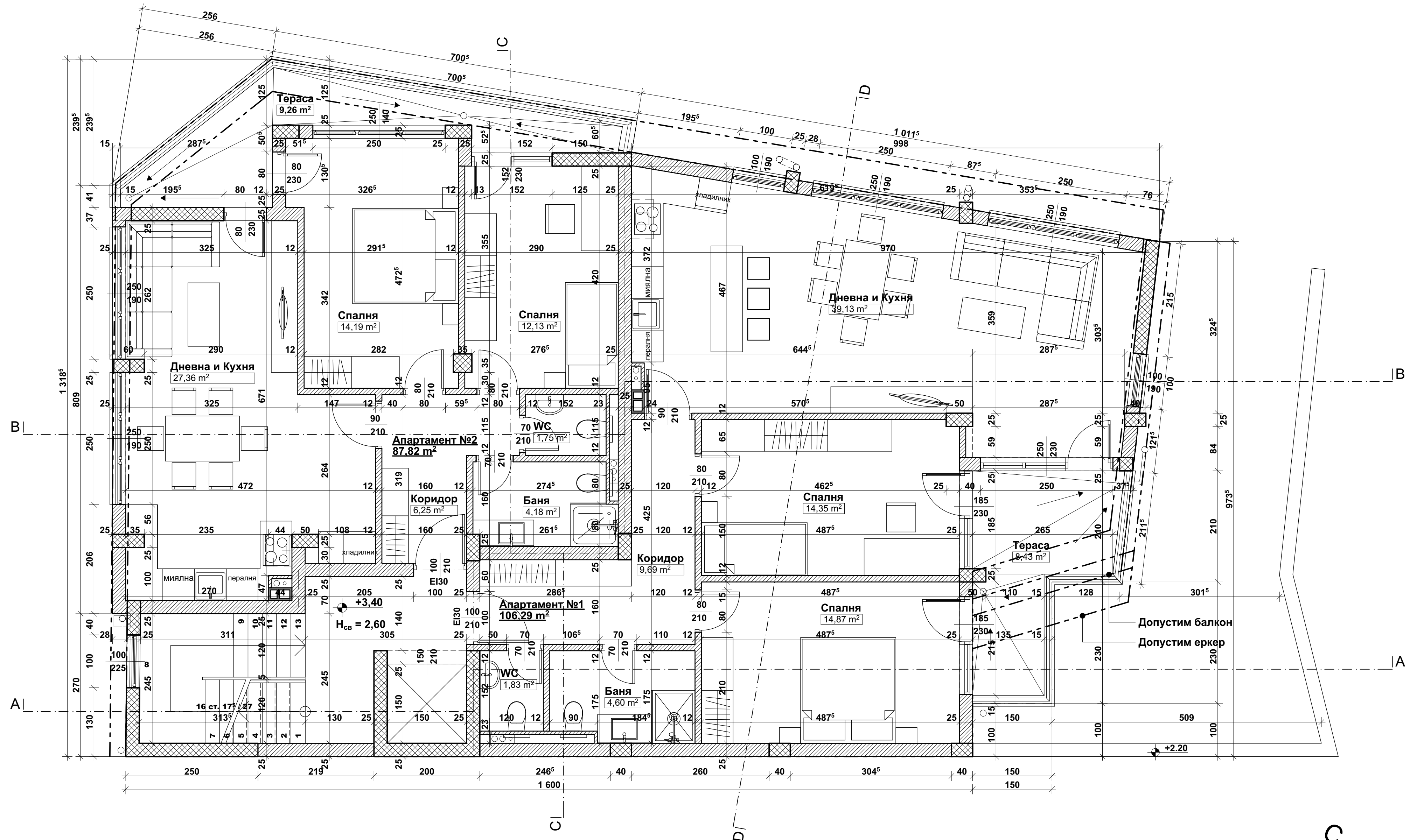
РАЗПРЕДЕЛЕНИЕ ПЪРВИ ЕТАЖ М 1:50 ЗП - 216,07 m 2
