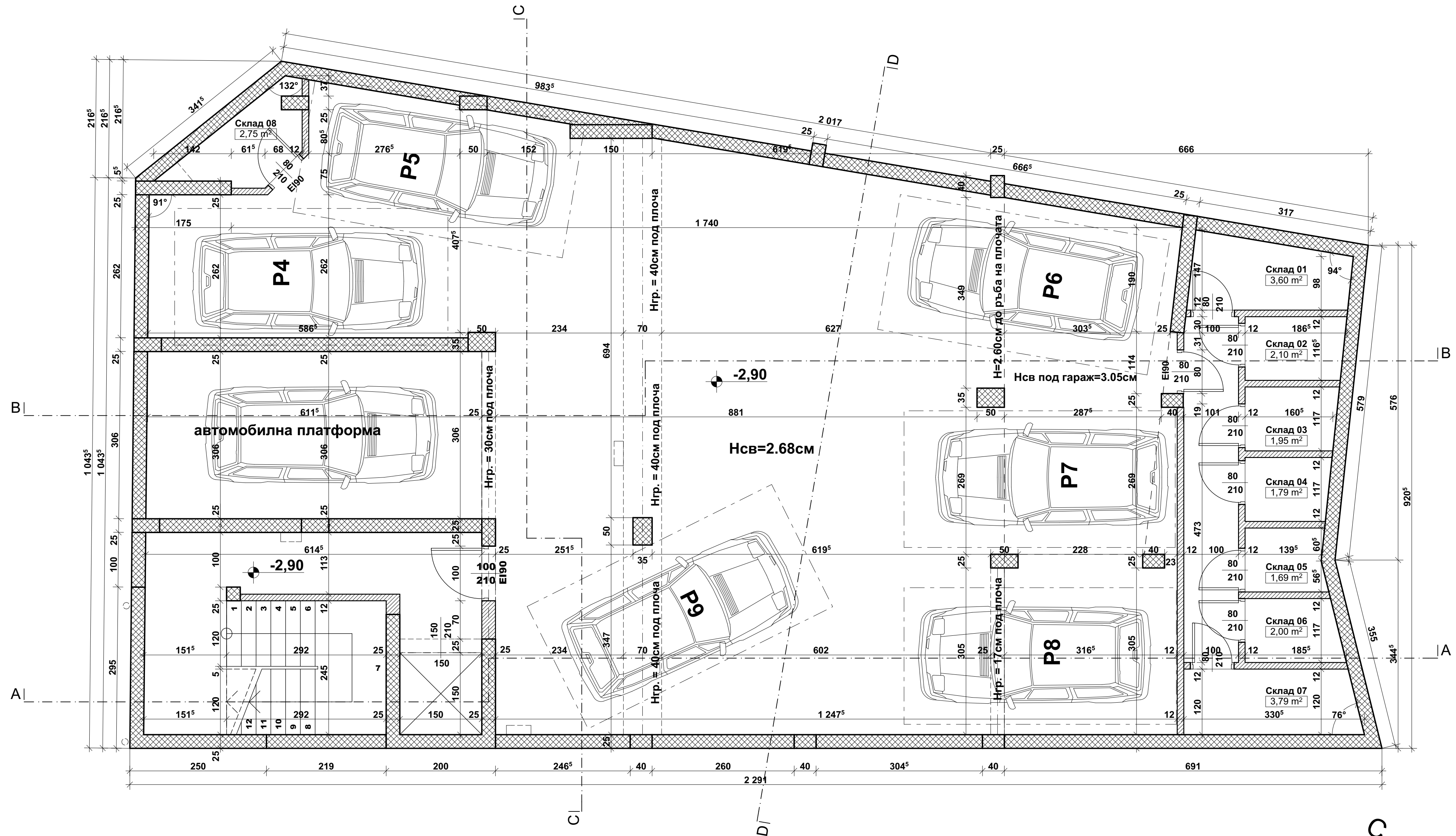
РАЗПРЕДЕЛЕНИЕ СУТЕРЕН М 1:50 ЗП - 245,38 m 2
