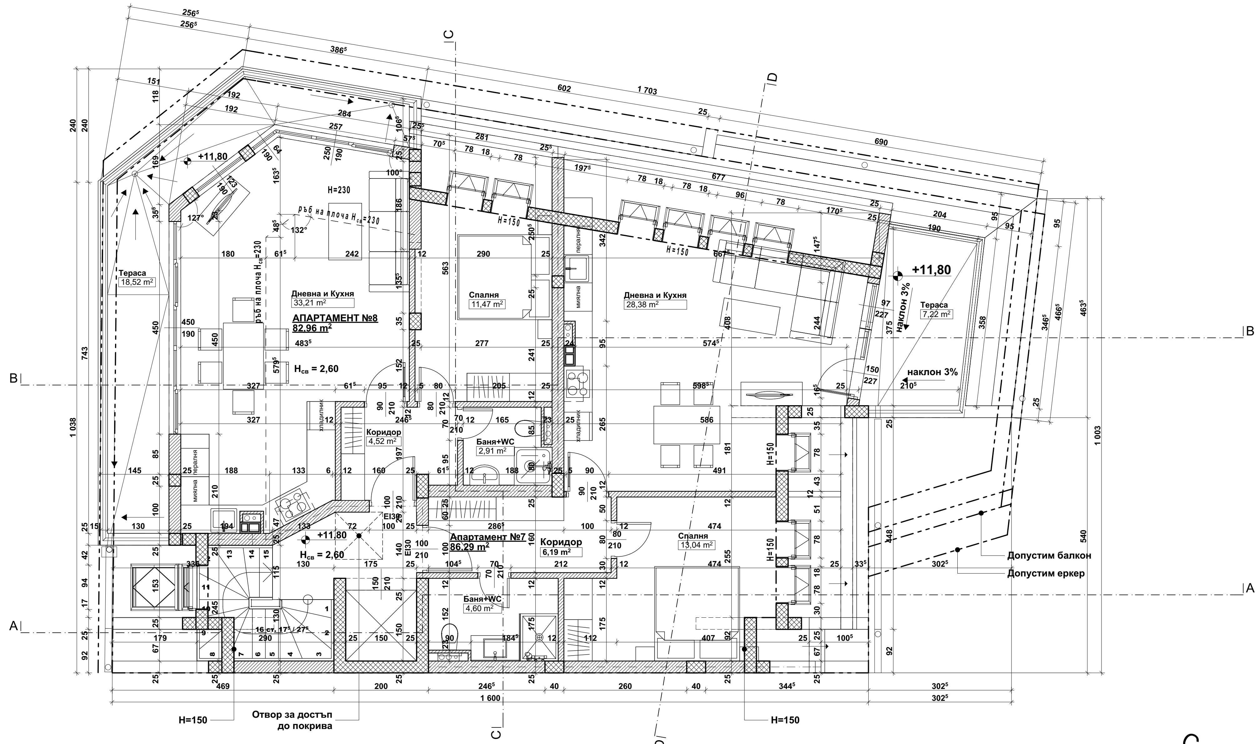
РАЗПРЕДЕЛЕНИЕ ПОДПОКРИВНО НИВО М 1:50 ЗП - 181,77 m²
