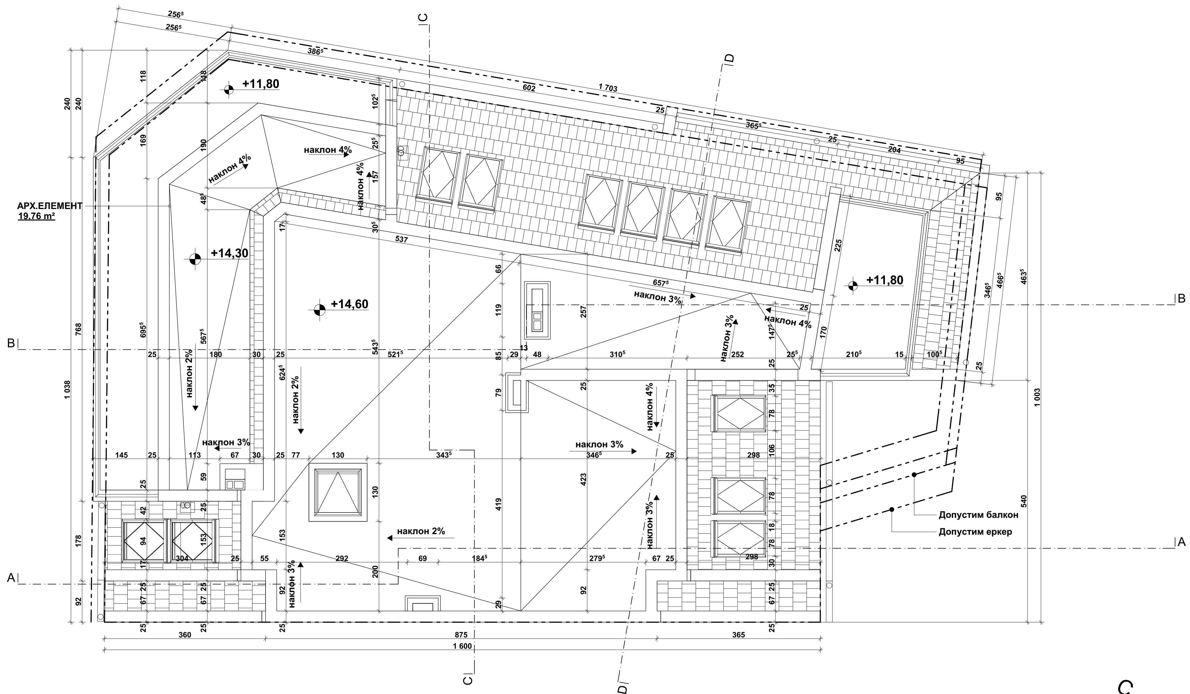
ПЛАН НА ПОКРИВА М 1:50
