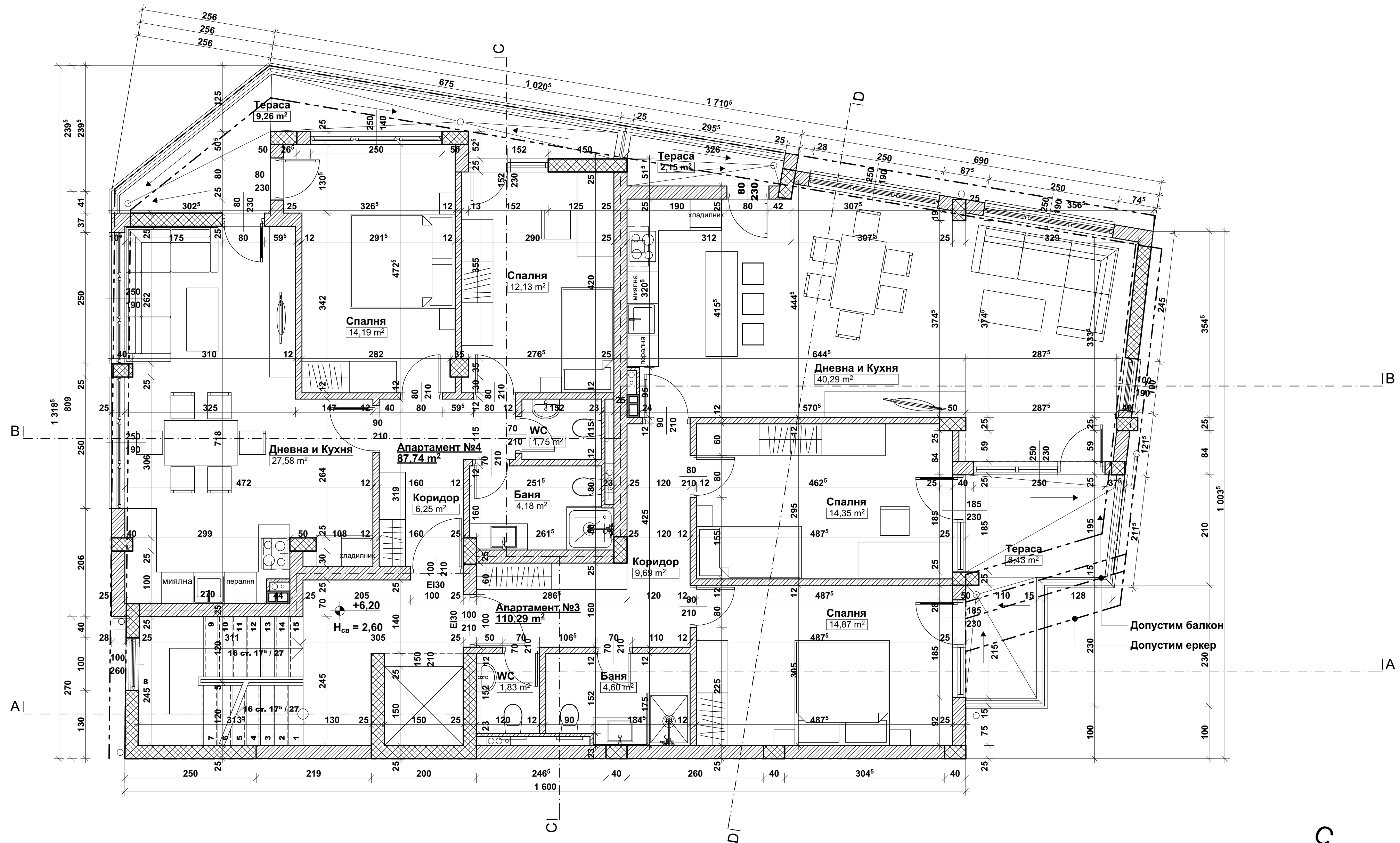
РАЗПРЕДЕЛЕНИЕ ВТОРИ ЕТАЖ М 1:50 ЗП - 220,03 m²
