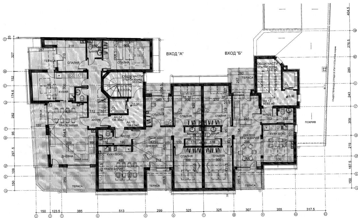
РАЗПРЕДЕЛЕНИЕ ниво 13.90 - Тавански ЕТАЖ м 1:150
