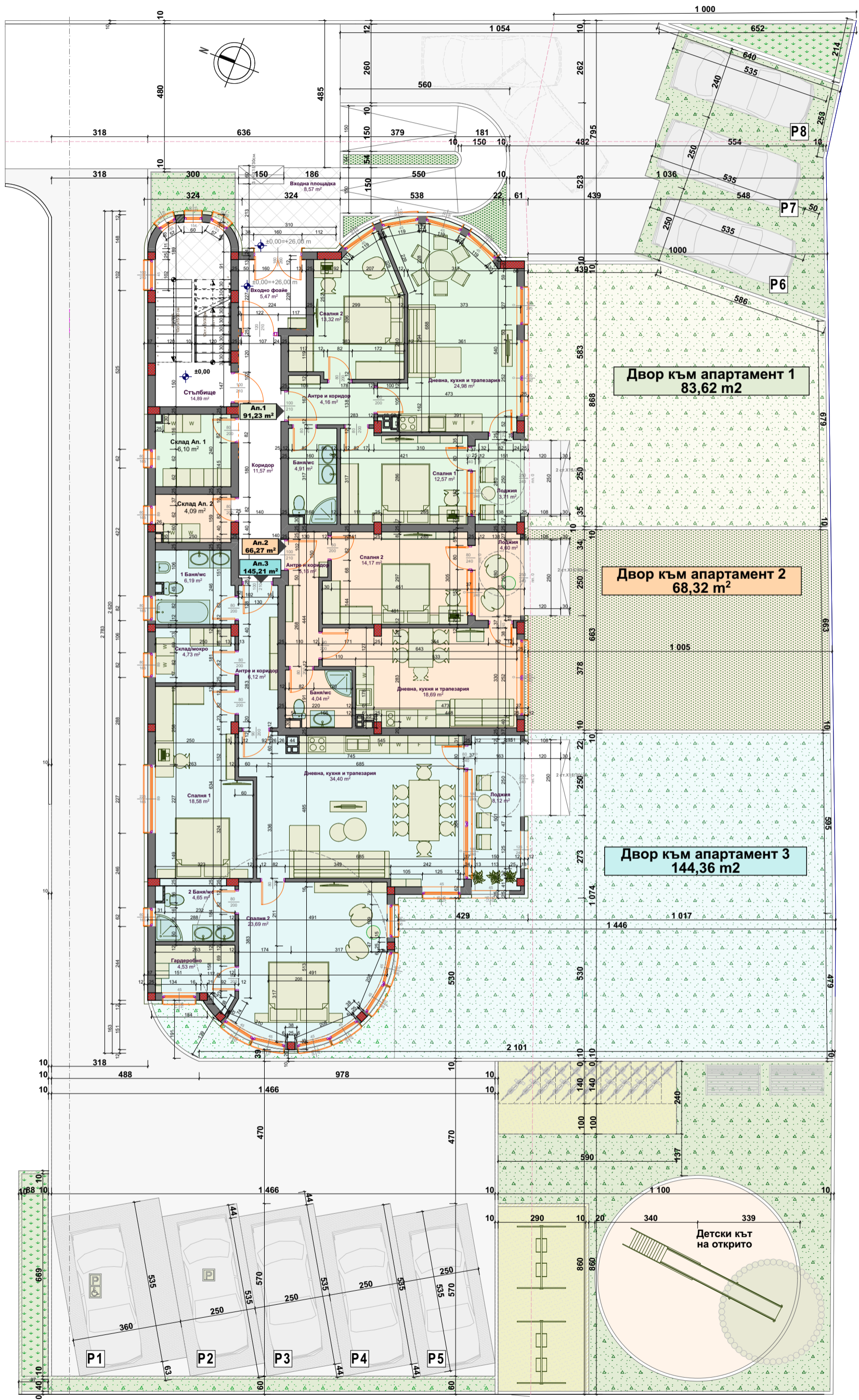
Жилищна сграда с апартаменти за гости - План партер
