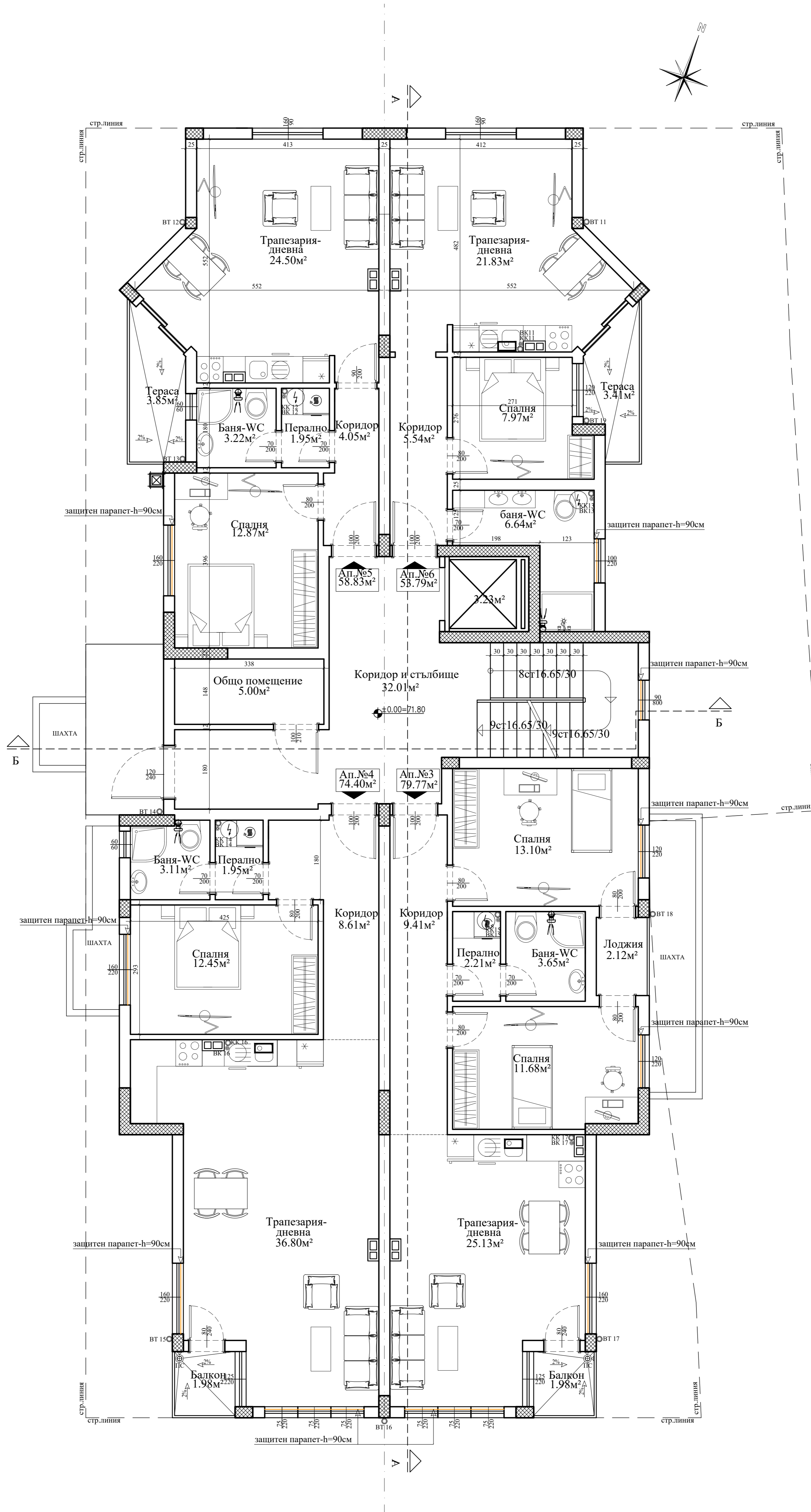
РАЗПРЕДЕЛЕНИЕ ПЪРВИ ЕТАЖ КОТА ±0.00
