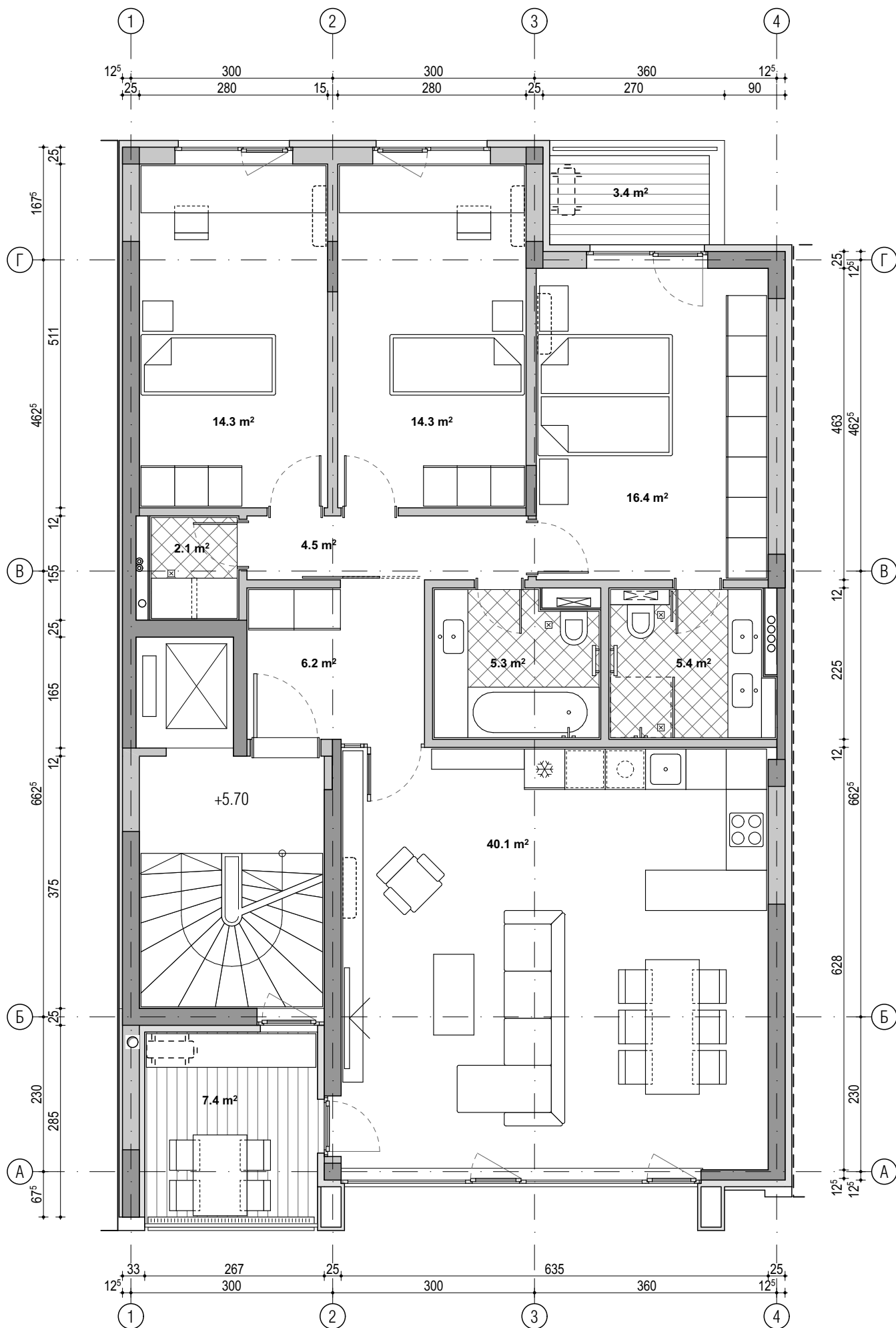
РАЗПРЕДЕЛЕНИЕ ЭТАЖ 3 (М1:75)
