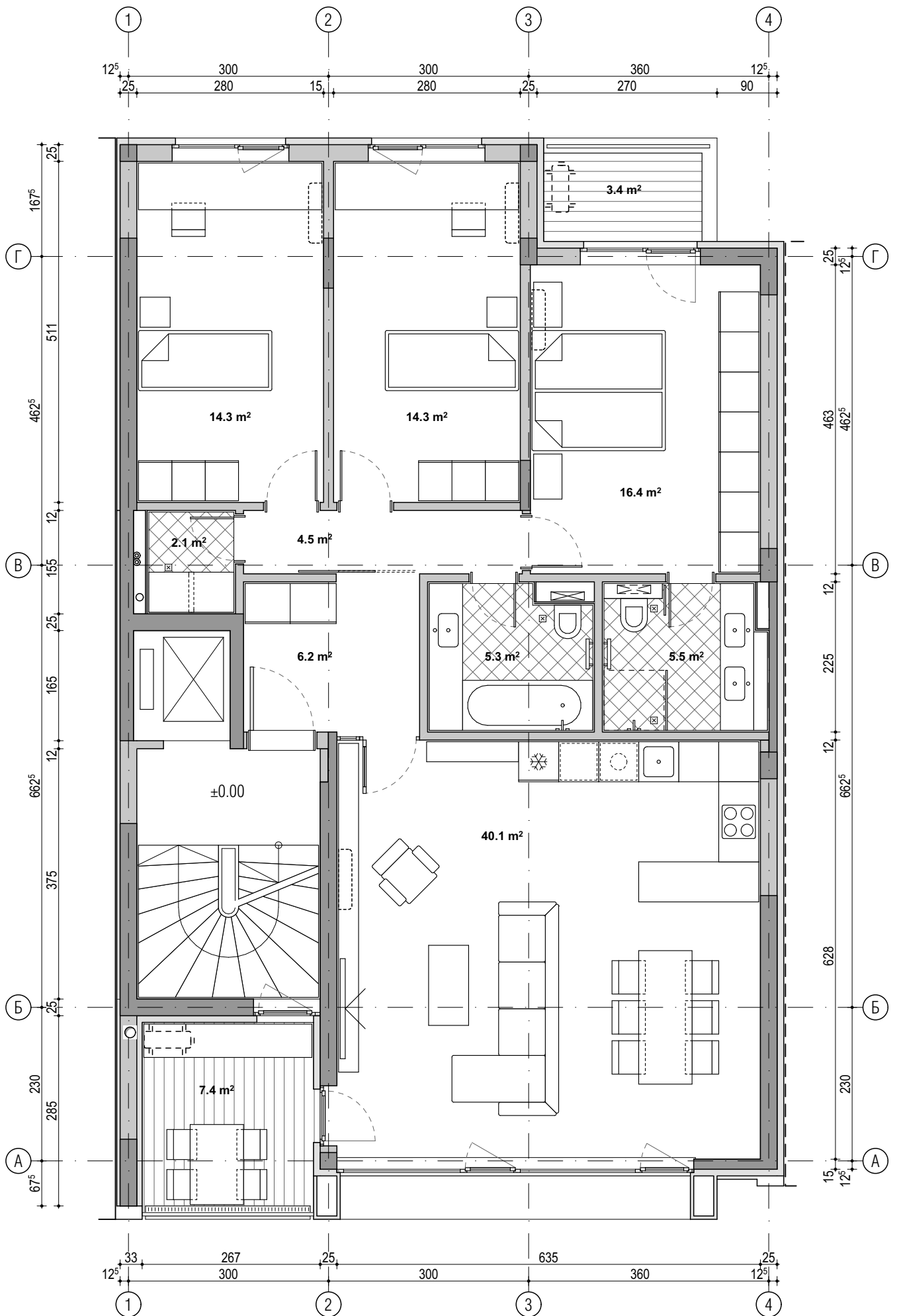
РАЗПРЕДЕЛЕНИЕ ЭТАЖ 1 (М1:75)
